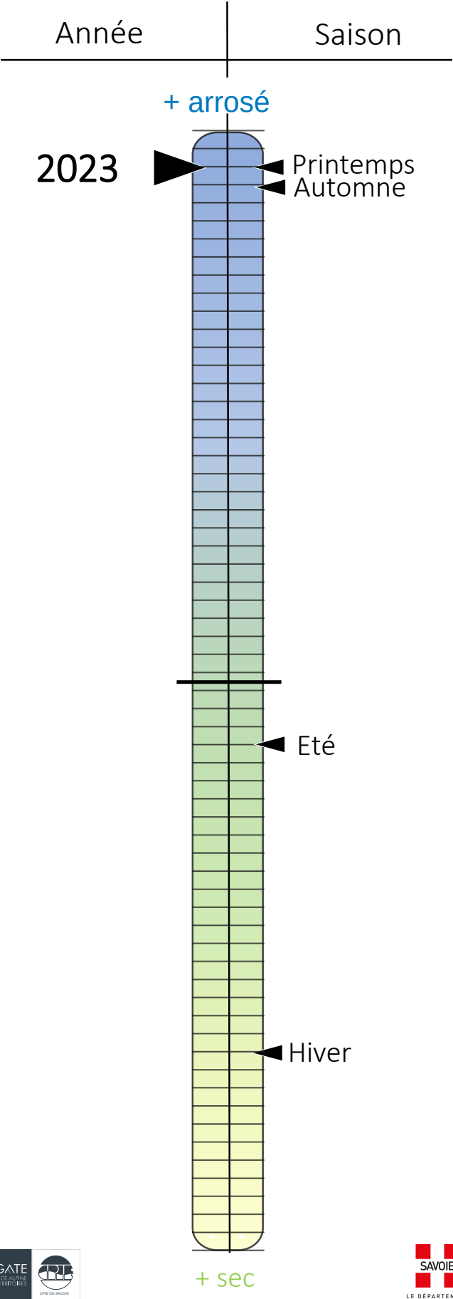
Écarts des cumuls moyens annuelles de précipitations (en mm) par rapport à la normale 1961-1990 de 1959 à 2023 dans les Alpes du Nord.
