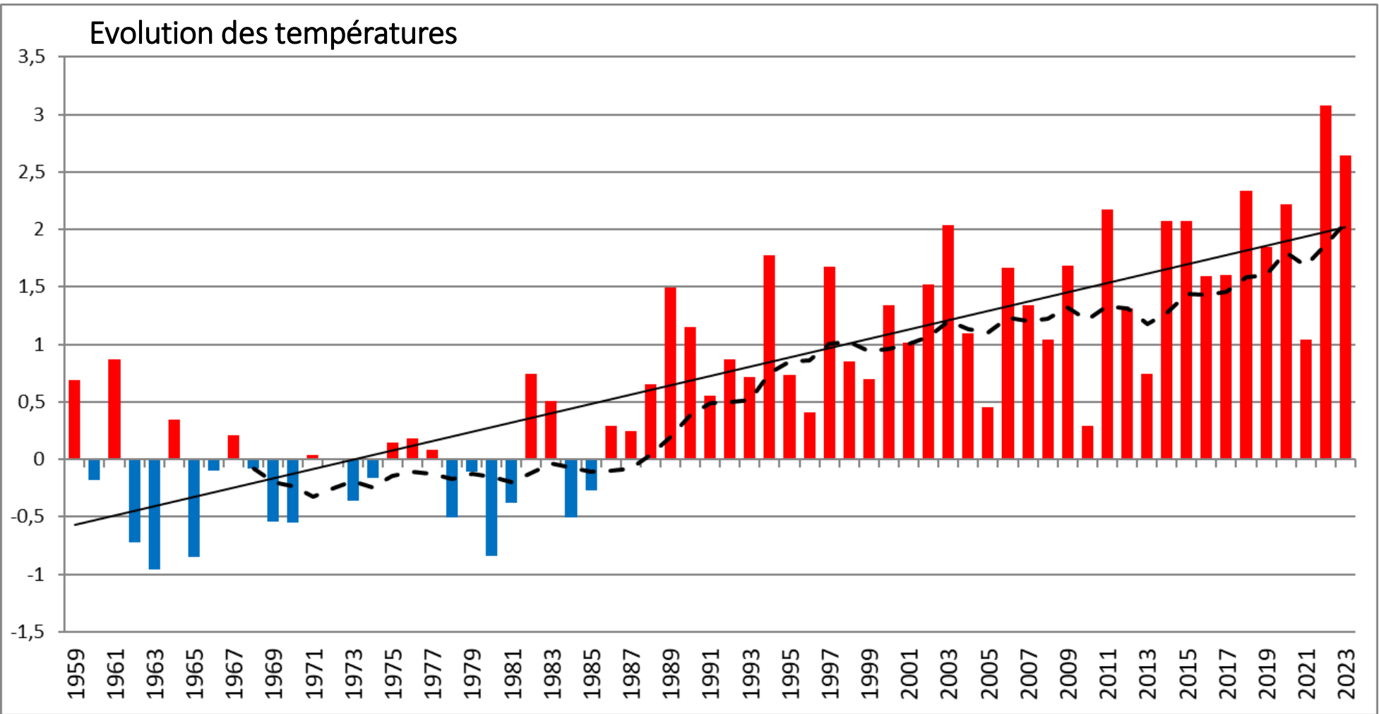
Écarts des températures moyennes annuelles (en °C) par rapport à la normale 1961-1990 de 1959 à 2023 dans les Alpes du Nord.
