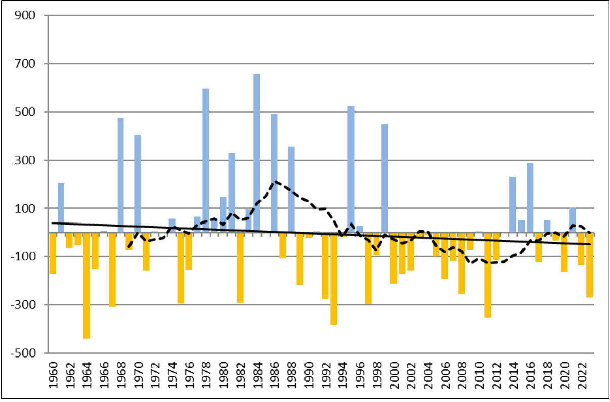
Écarts des cumuls de neige en cm de l'avant-saison (nov-déc, graphique de gauche), de la pleine saison (janv-fev, au centre) et de l'arrière-saison (mars-avril, à droite) de 1959 à 2023 par rapport à la normale 1961-1990 dans les Alpes du Nord
