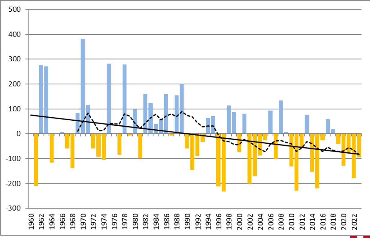
Écarts des cumuls de neige en cm de l'avant-saison (nov-déc, graphique de gauche), de la pleine saison (janv-fev, au centre) et de l'arrière-saison (mars-avril, à droite) de 1959 à 2023 par rapport à la normale 1961-1990 dans les Alpes du Nord
