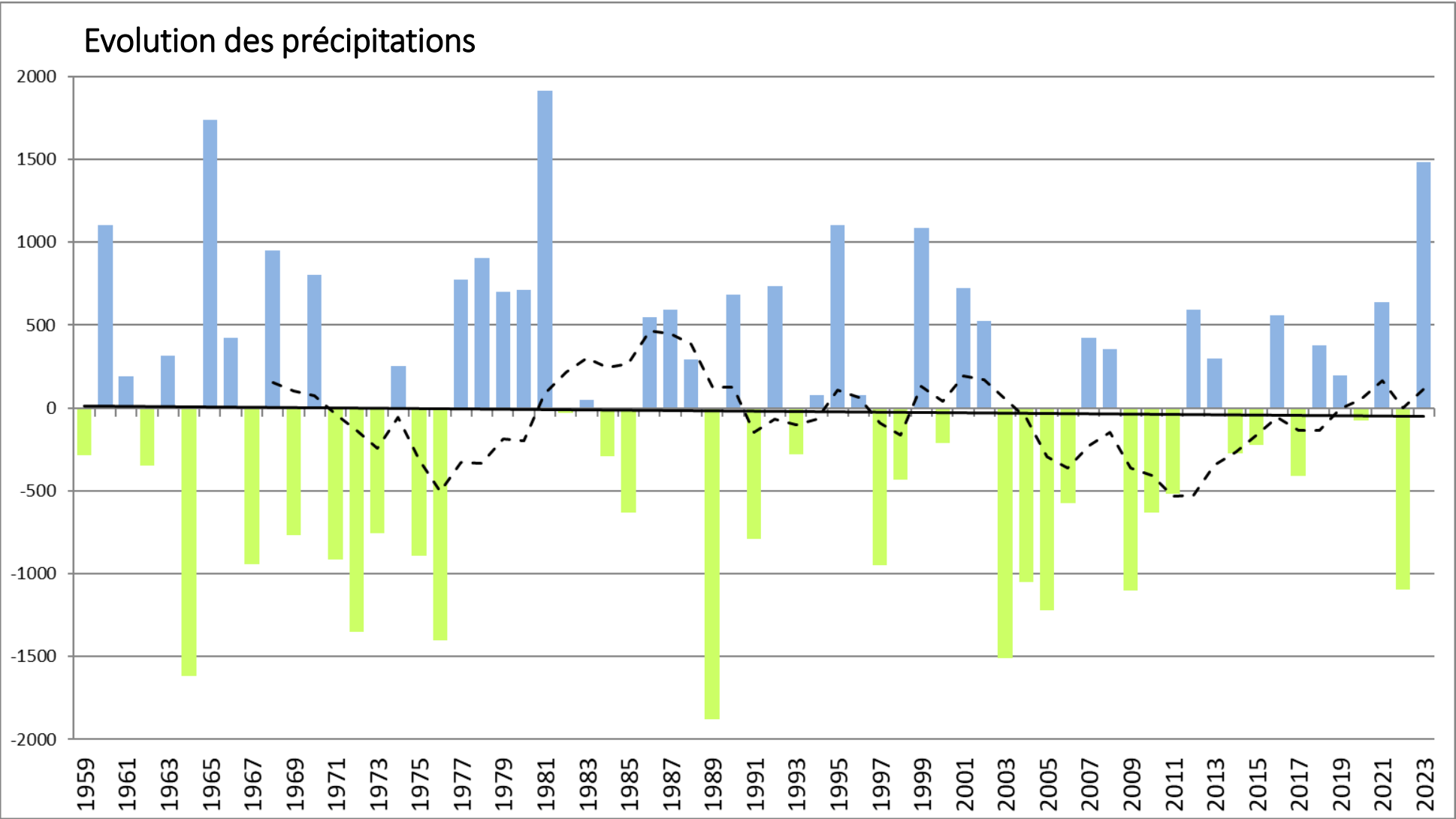
Écarts des cumuls moyens annuelles de précipitations (en mm) par rapport à la normale 1961-1990 de 1959 à 2023 dans les Alpes du Nord.
